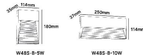
W48S-B-5W
